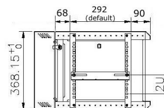
B-B
